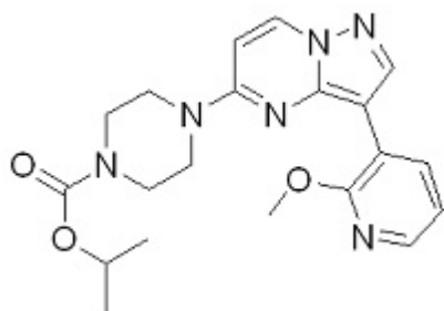
PC-6063501, CDCl 3
